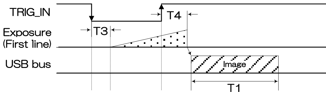
Level mode (Image format : all pixels readout)
