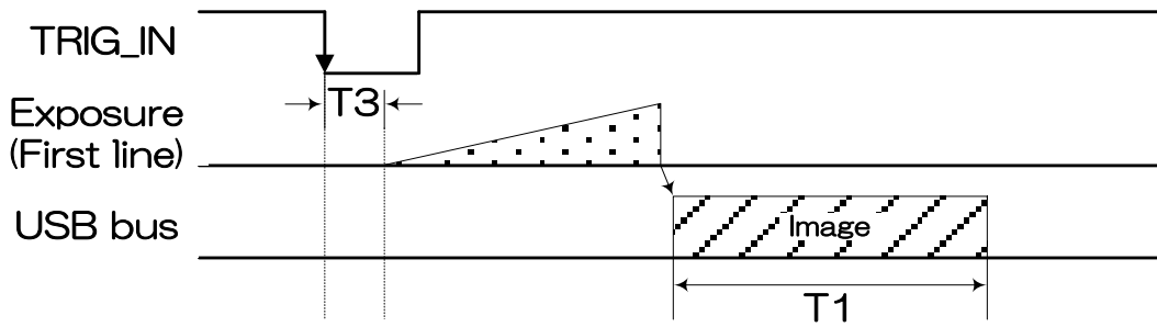
Edge mode (Image format : all pixels readout)
